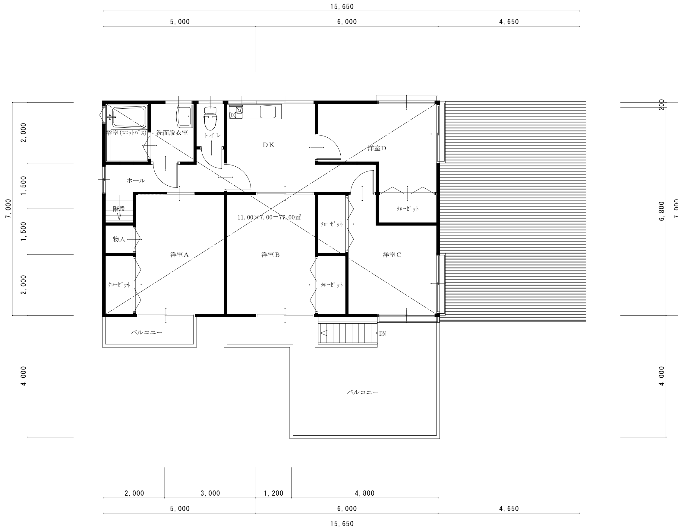
2階平面詳細図 SC1 : 75
